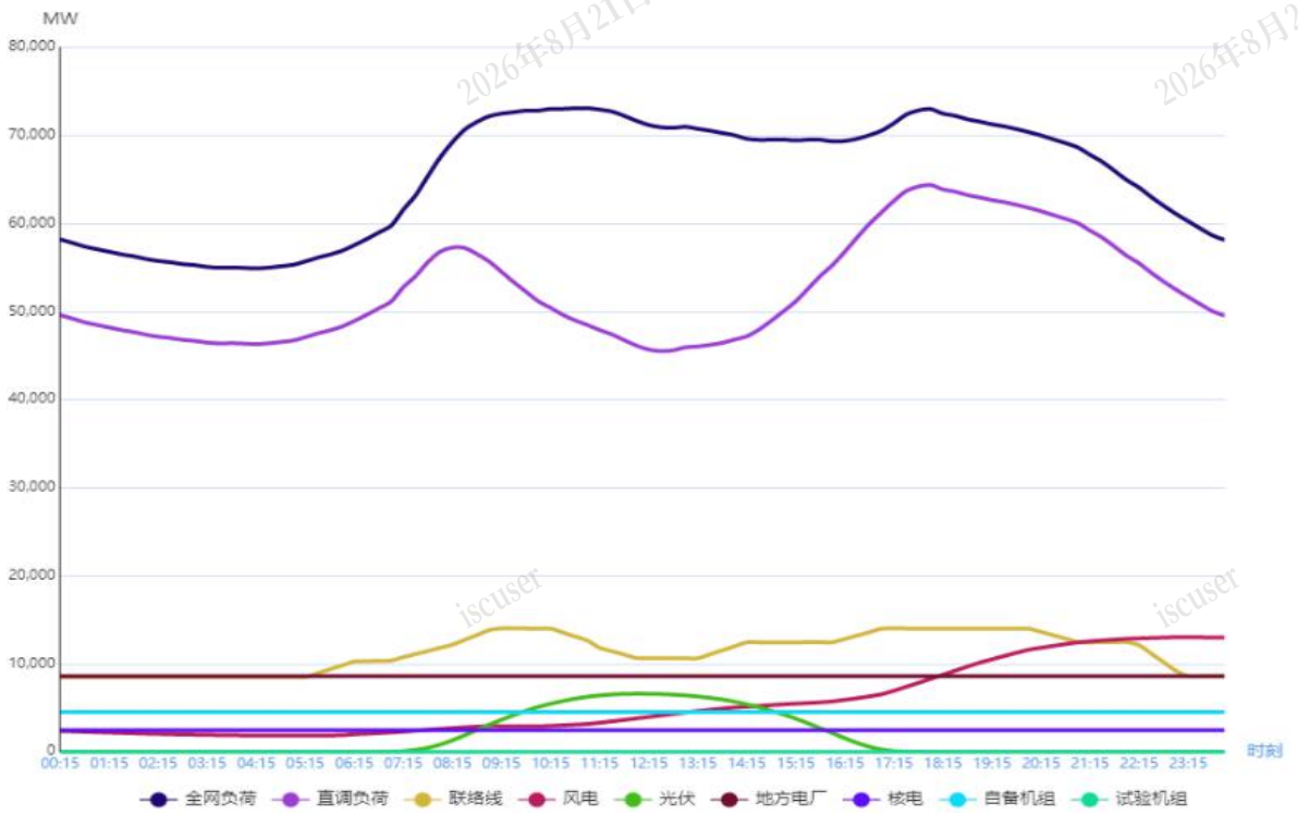
图1 1月18日负荷及电源出力预测情况
