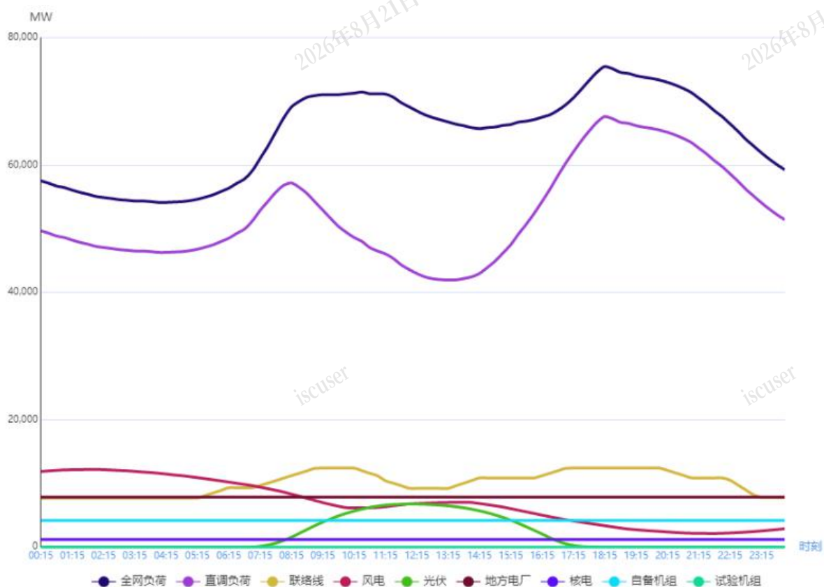
图 1 1 月 29 日负荷及电源出力预测情况
