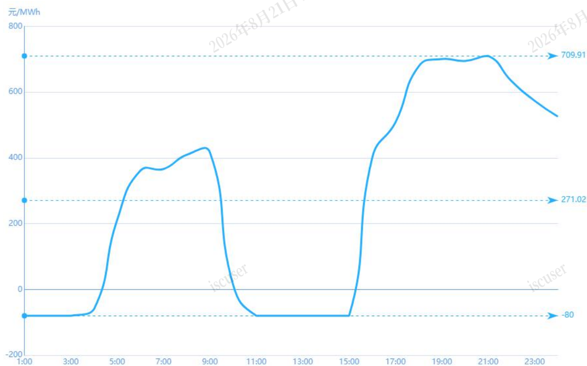
图3 1月29日实时市场用电侧价格
