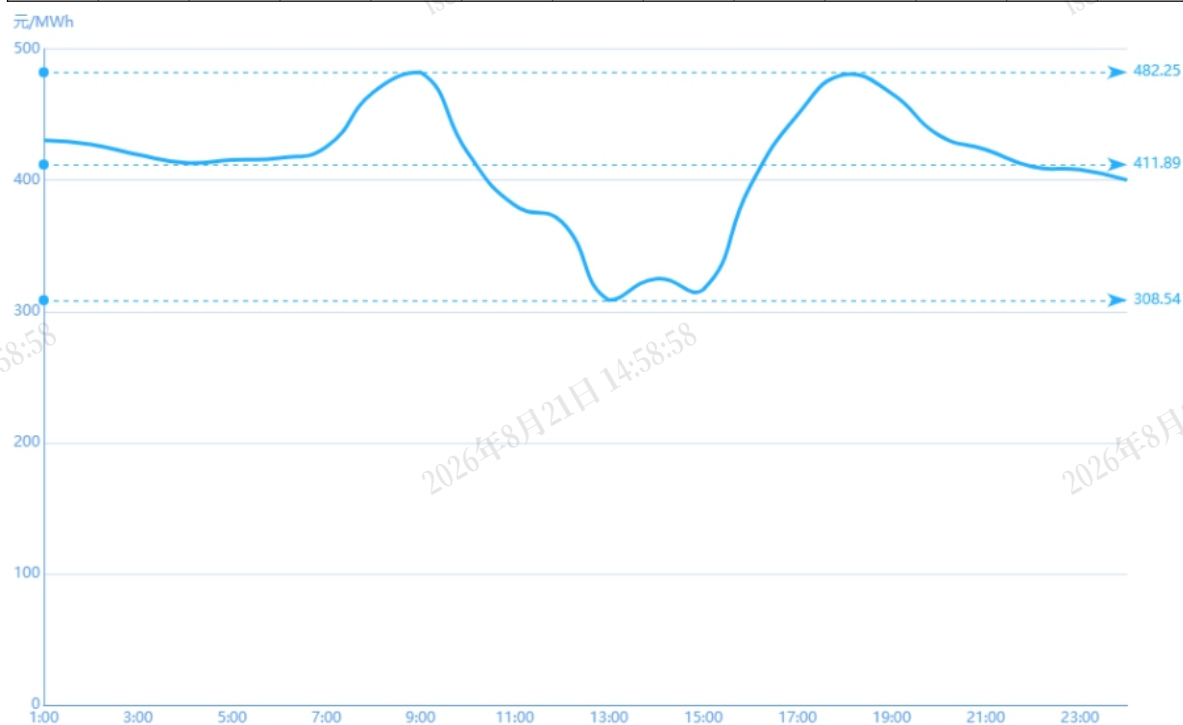
图 3 2月4日实时市场用电侧价格
