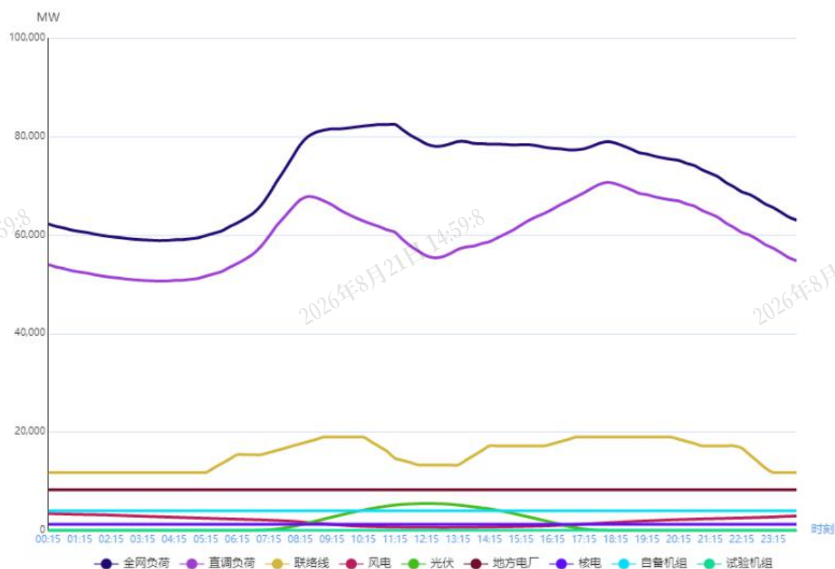
图 1 2月7日负荷及电源出力预测情况
