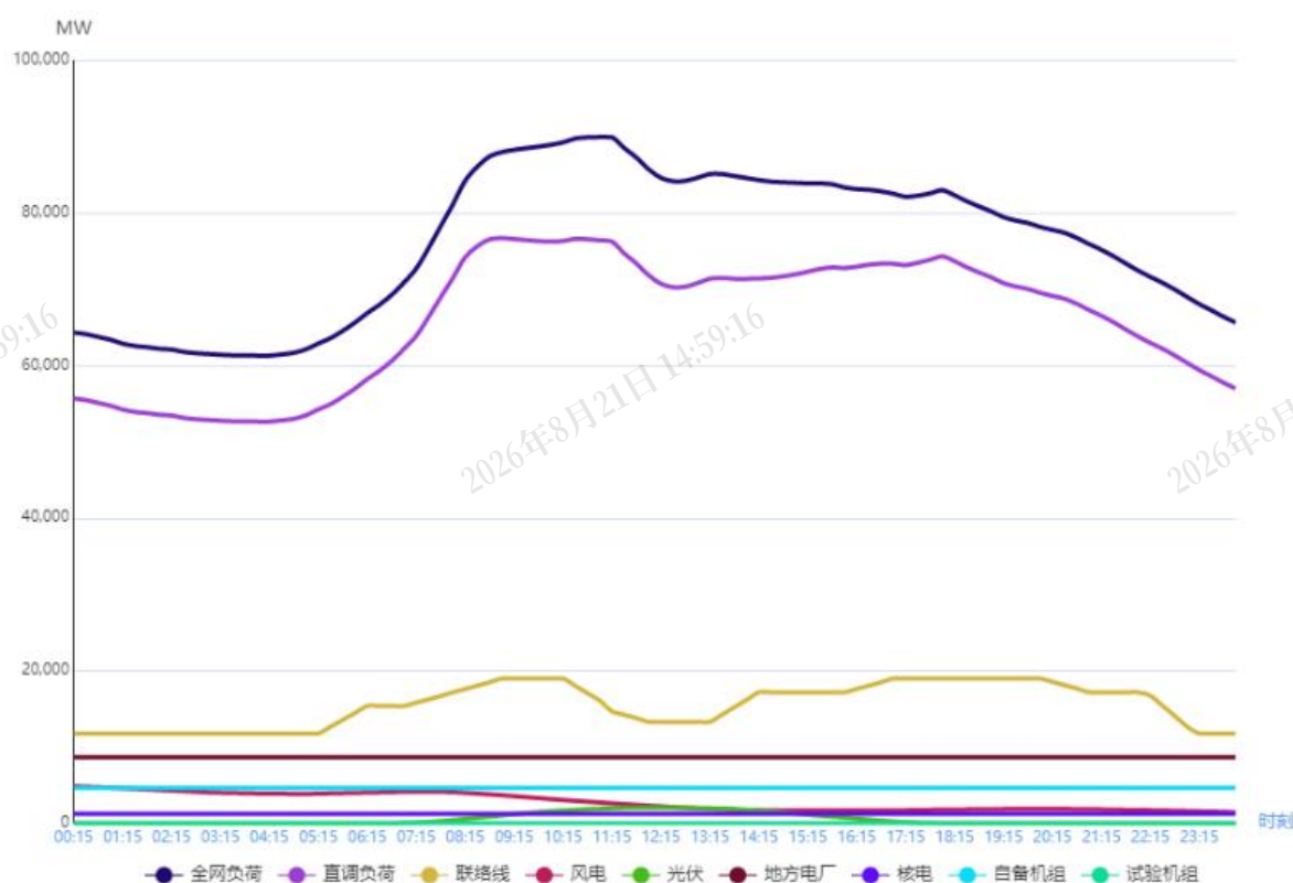
图1 2月9日负荷及电源出力预测情况
