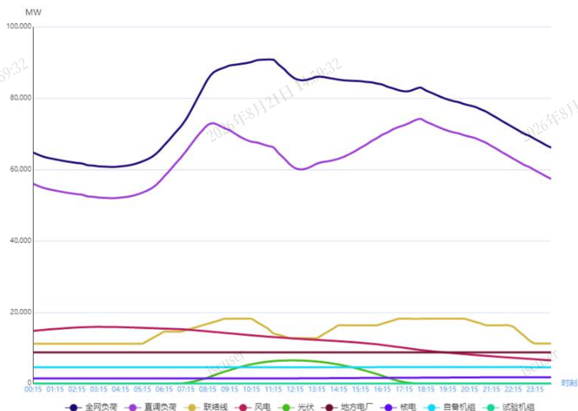
图 1 2月13日负荷及电源出力预测情况
