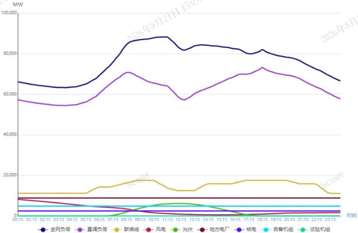
图 1 2月23日负荷及电源出力预测情况
