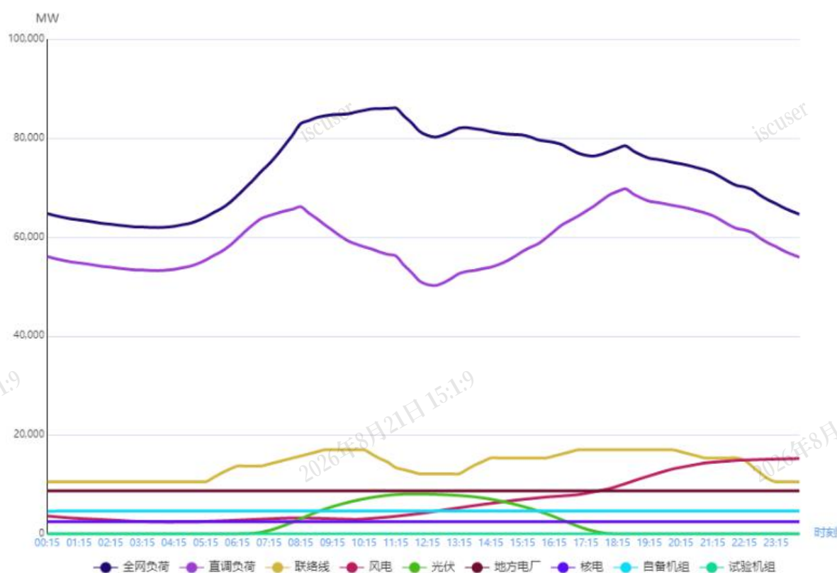
图1 3月2日负荷及电源出力预测情况
