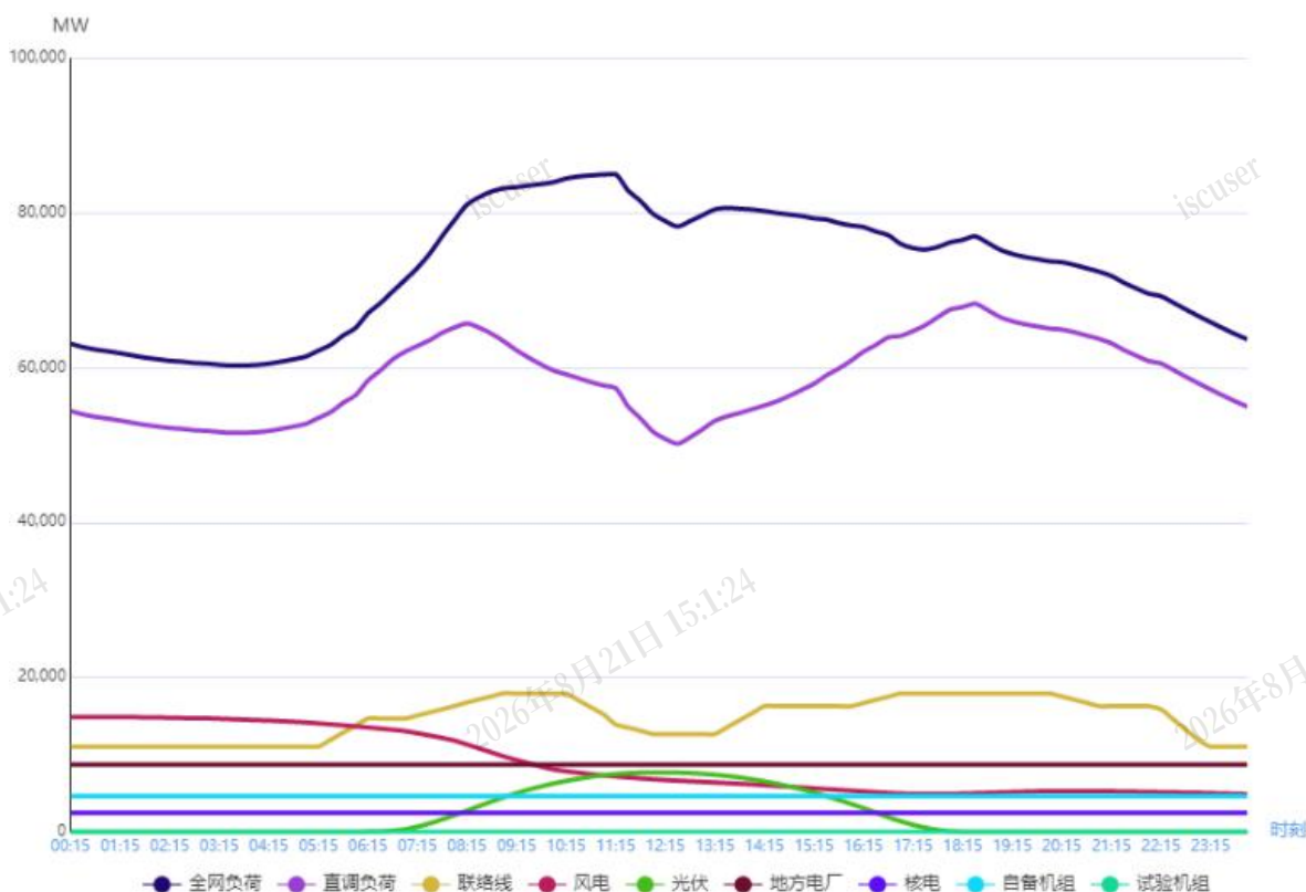
图1 3月6日负荷及电源出力预测情况
