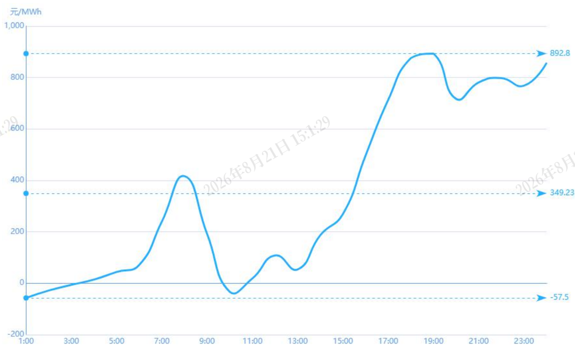
图 3 3月6日实时市场用电侧价格
