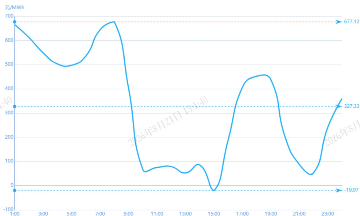
图 3 3月9日实时市场用电侧价格
