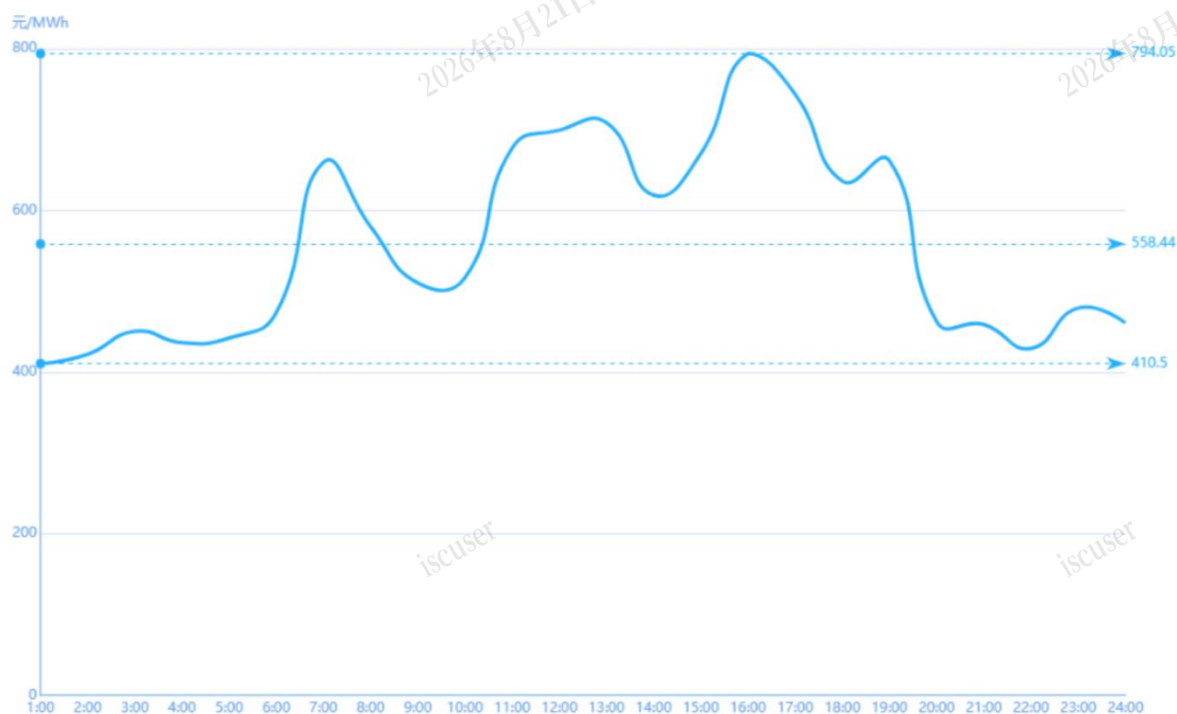
图3 3月16日实时市场用电侧价格
