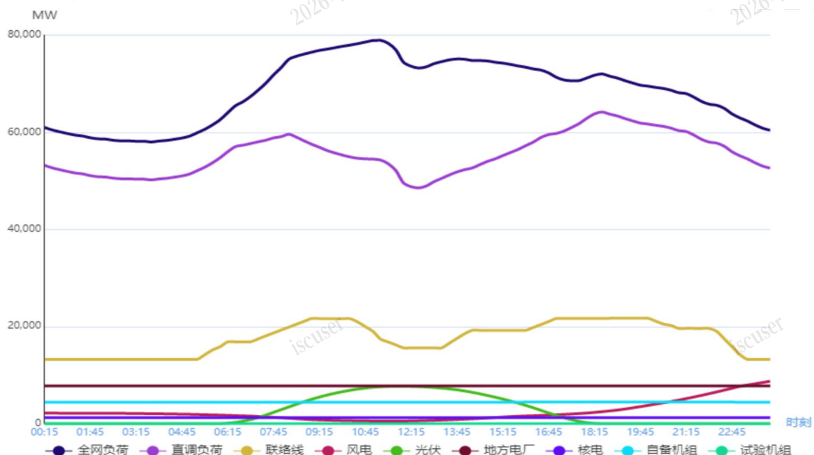
图 1 3月26日负荷及电源出力预测情况
