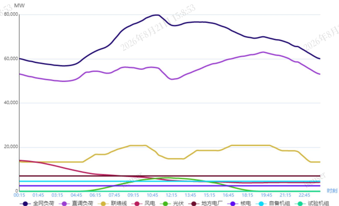
图1 5月20日负荷及电源出力预测情况
