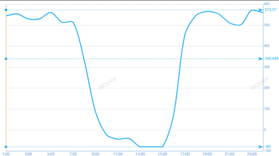
图2 6月1日日前市场用电侧价格
