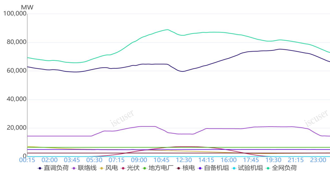
图 1 6月29日负荷及电源出力预测情况
