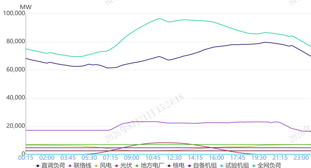
图1 7月10日负荷及电源出力预测情况
