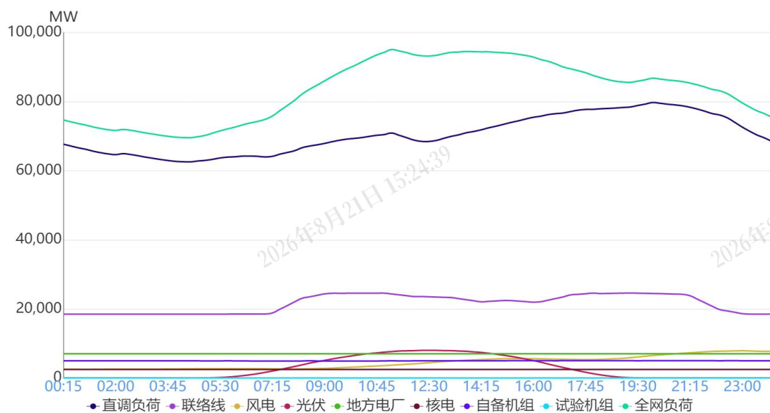
图1 7月14日负荷及电源出力预测情况
