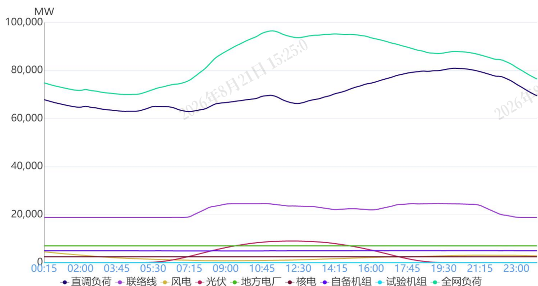
图1 7月18日负荷及电源出力预测情况
