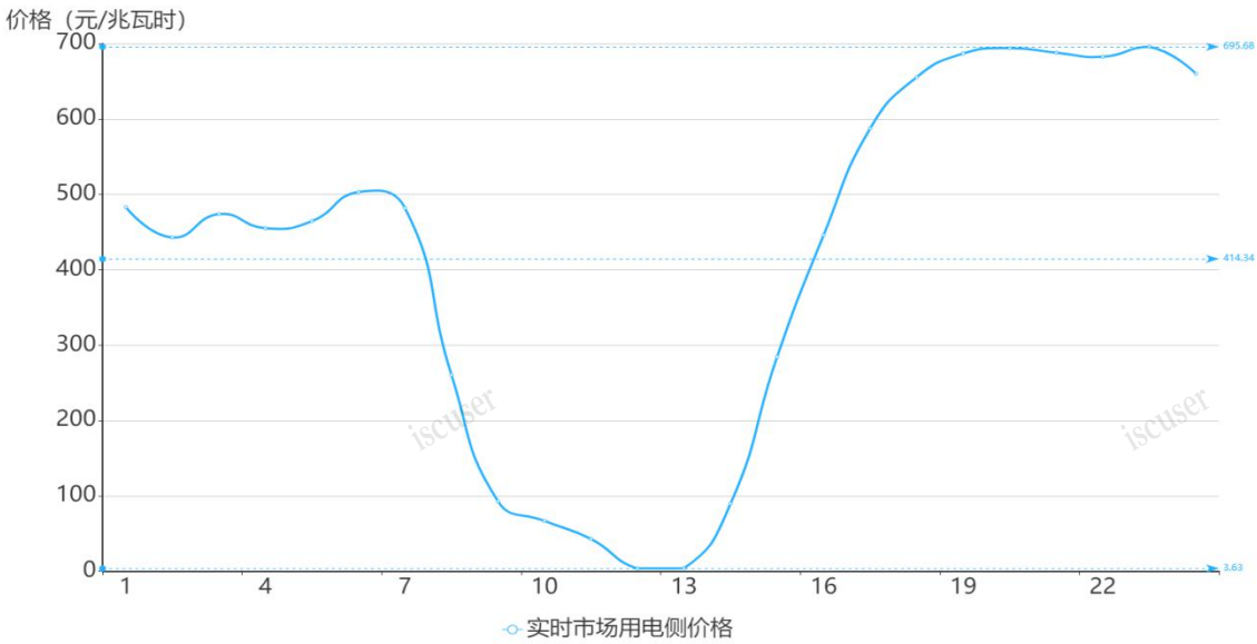
图 3 7 月 17 日实时市场用电侧价格
