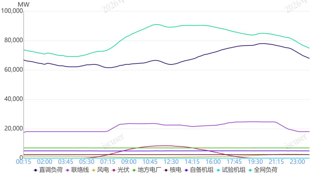
图 1 7月23日负荷及电源出力预测情况
