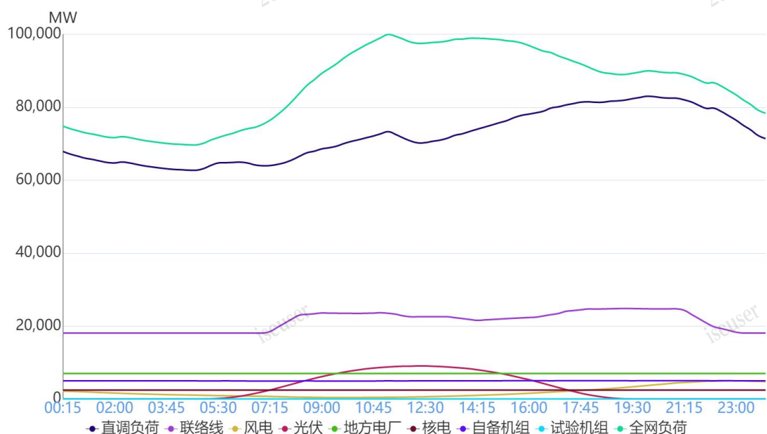
图 1 7月24日负荷及电源出力预测情况
