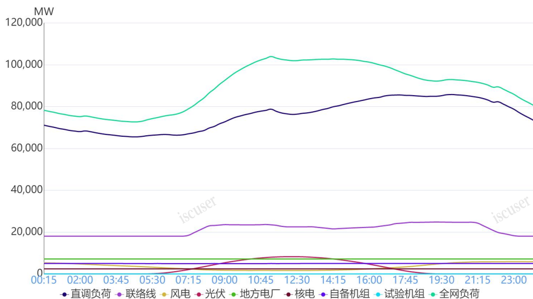
图 1 7月25日负荷及电源出力预测情况
