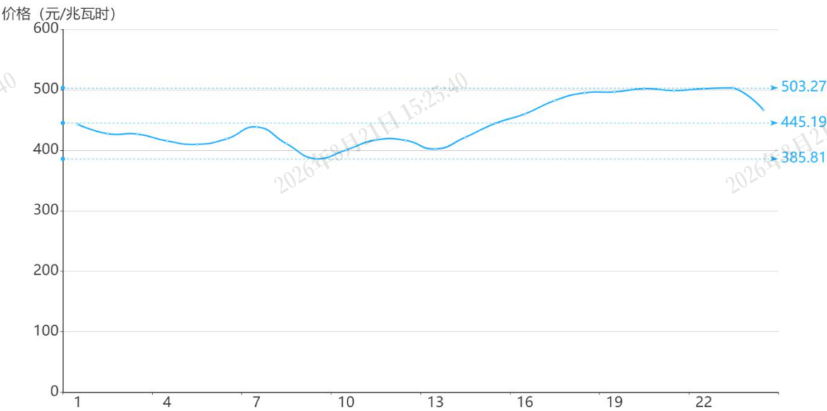
图 2 7 月 27 日日前市场用电侧价格
