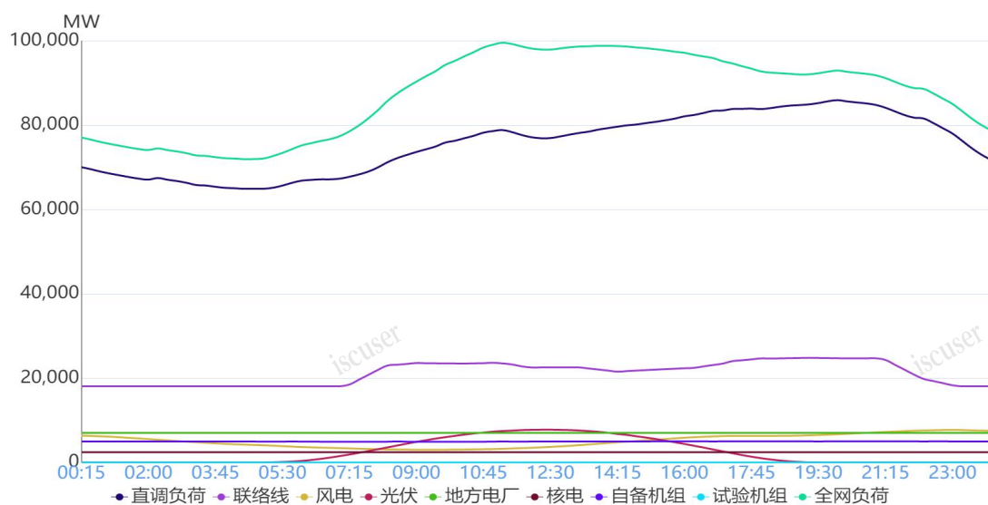
图 1 7月27日负荷及电源出力预测情况
