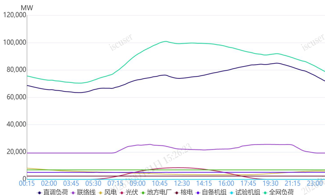
图 1 8月1日负荷及电源出力预测情况
