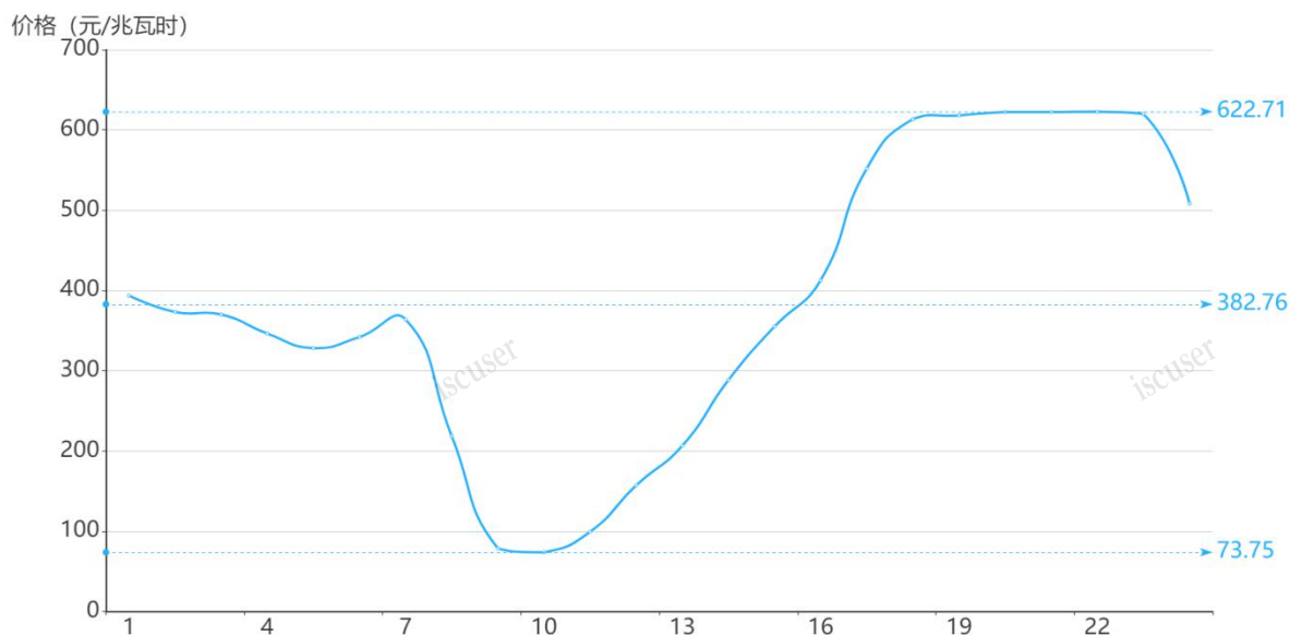
图2 8月1日日前市场用电侧价格
