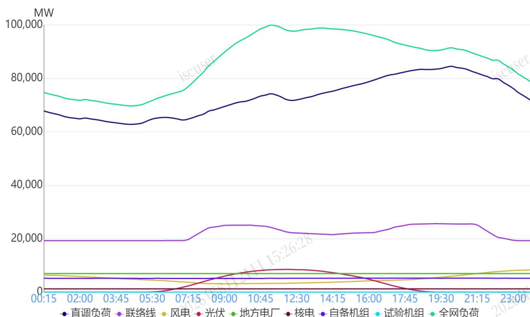
图 1 8月2日负荷及电源出力预测情况
