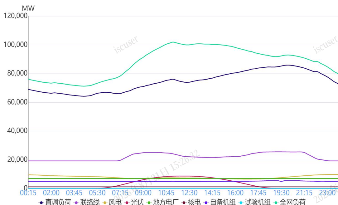
图 1 8月3日负荷及电源出力预测情况
