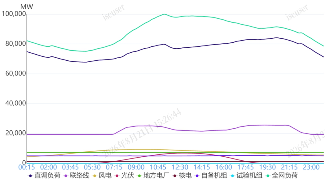
图 1 8月6日负荷及电源出力预测情况
