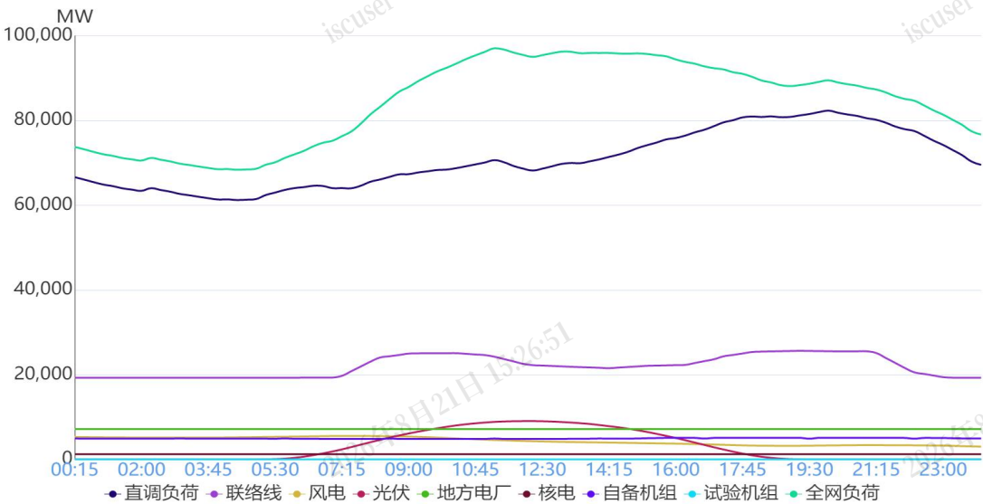
图 1 8月7日负荷及电源出力预测情况
