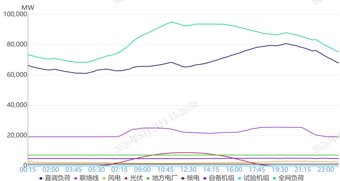
图 1 8月8日负荷及电源出力预测情况
