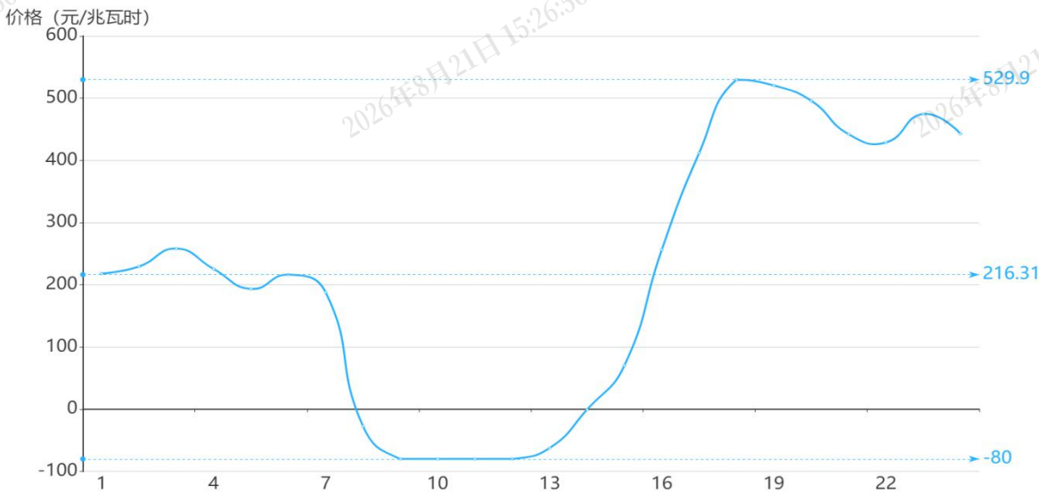
图 3 8 月 7 日实时市场用电侧价格
