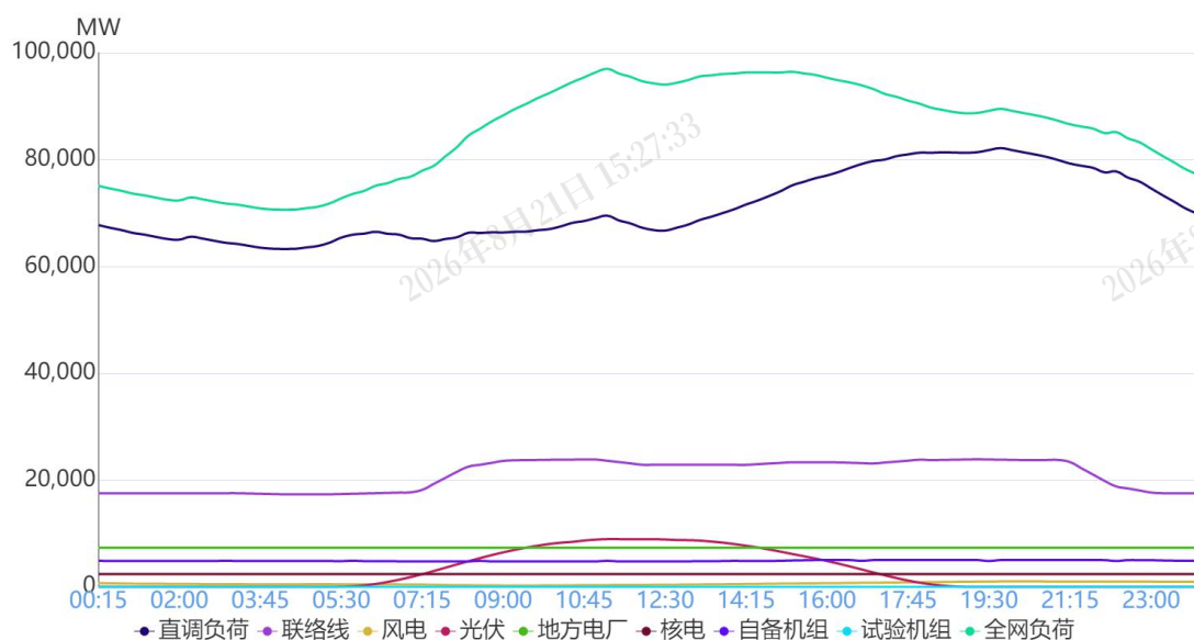
图1 8月15日负荷及电源出力预测情况
