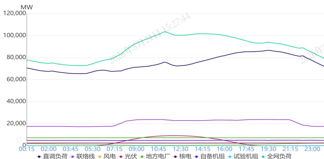
图 1 8月17日负荷及电源出力预测情况
