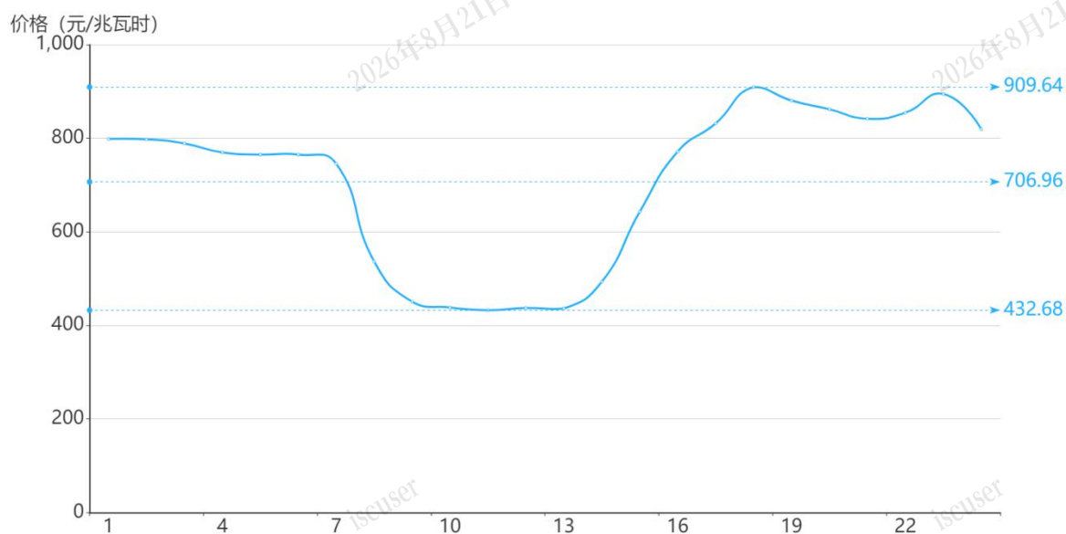
图3 8月17日实时市场用电侧价格
