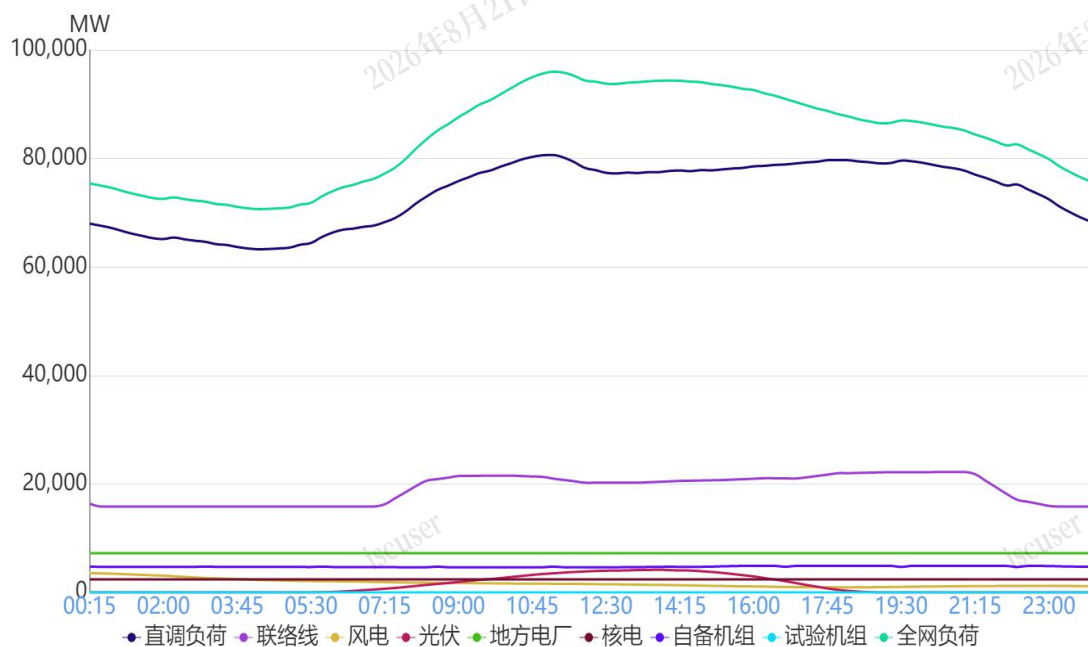
图 1 8月21日负荷及电源出力预测情况
