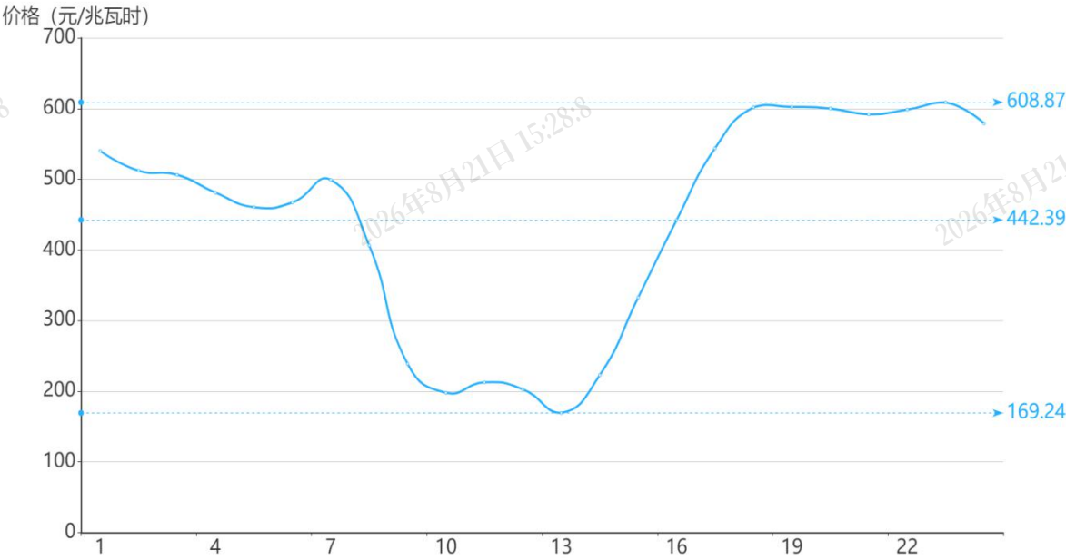
图 2 8 月 22 日日前市场用电侧价格
