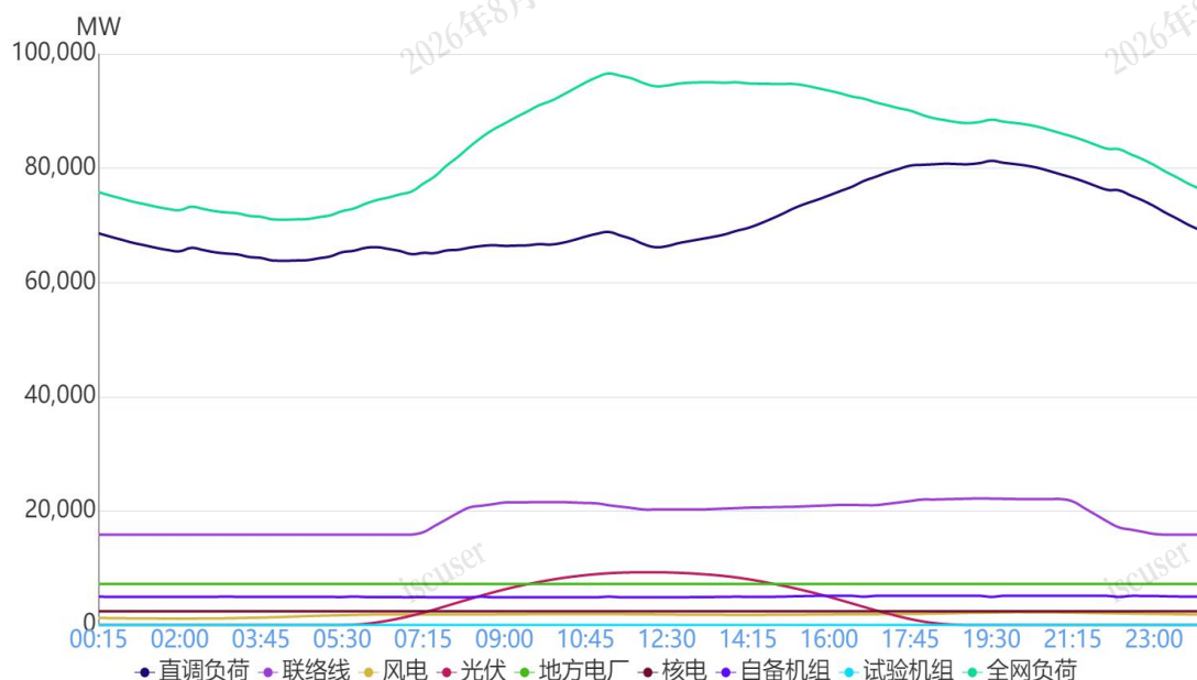
图 1 8月22日负荷及电源出力预测情况
