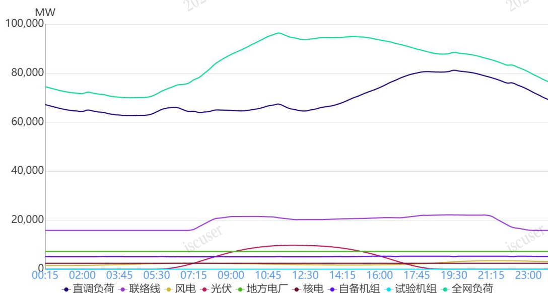
图 1 8月23日负荷及电源出力预测情况
