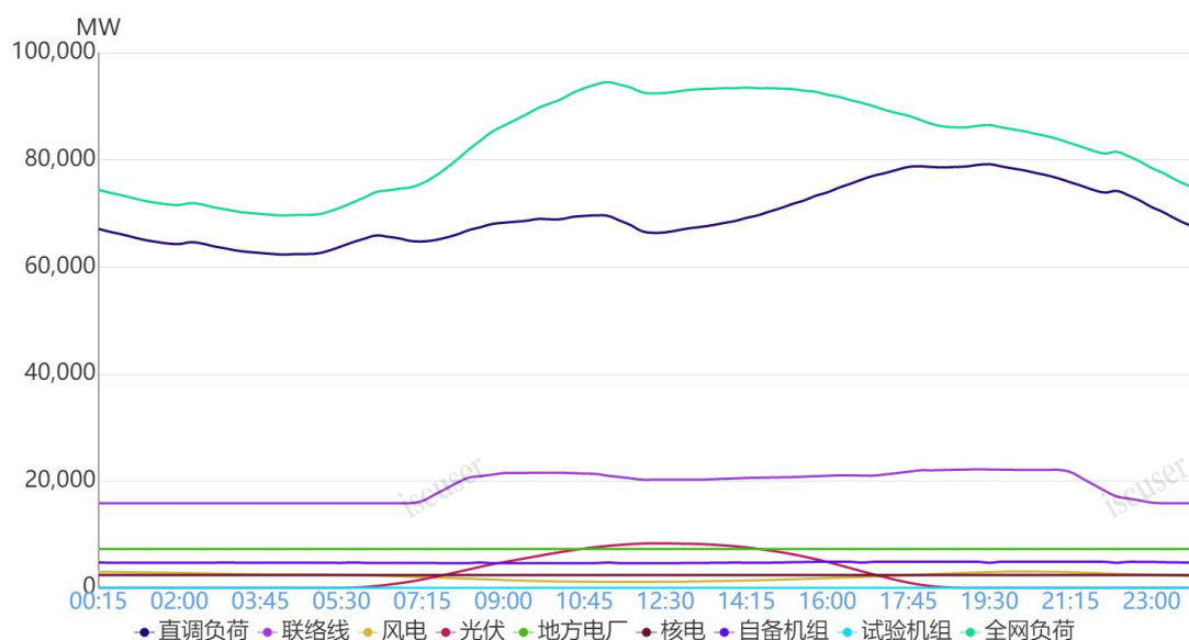
图 1 8月24日负荷及电源出力预测情况
