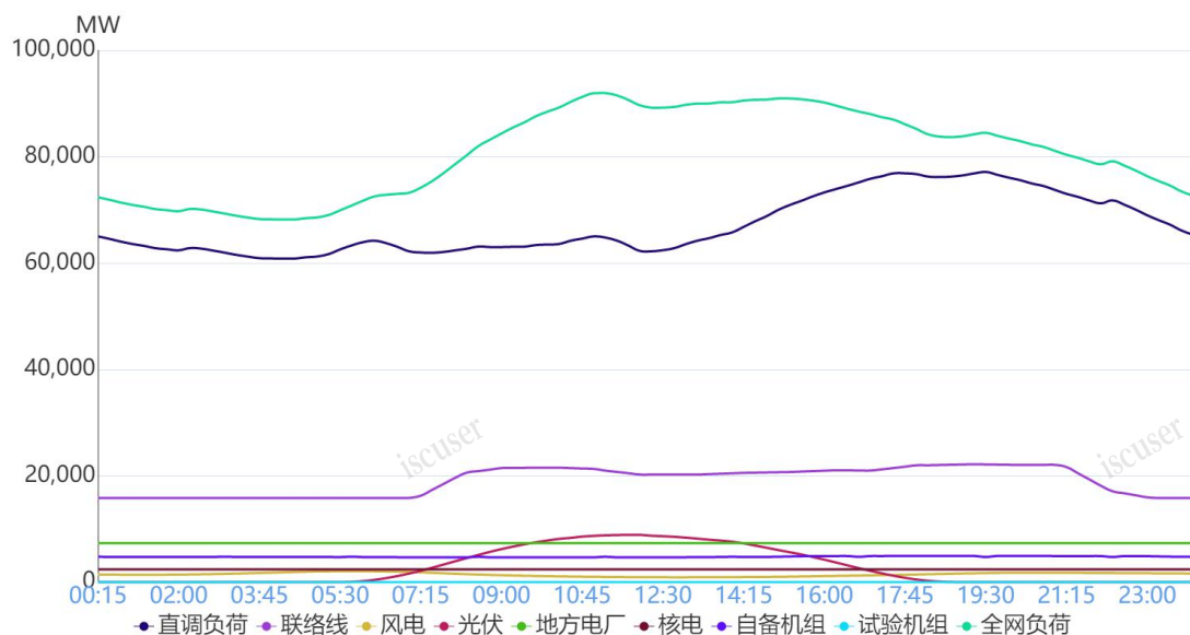
图1 8月25日负荷及电源出力预测情况
