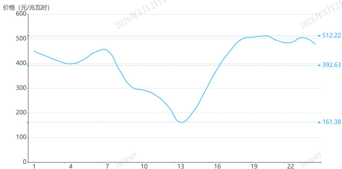
图 3 8 月 24 日实时市场用电侧价格
