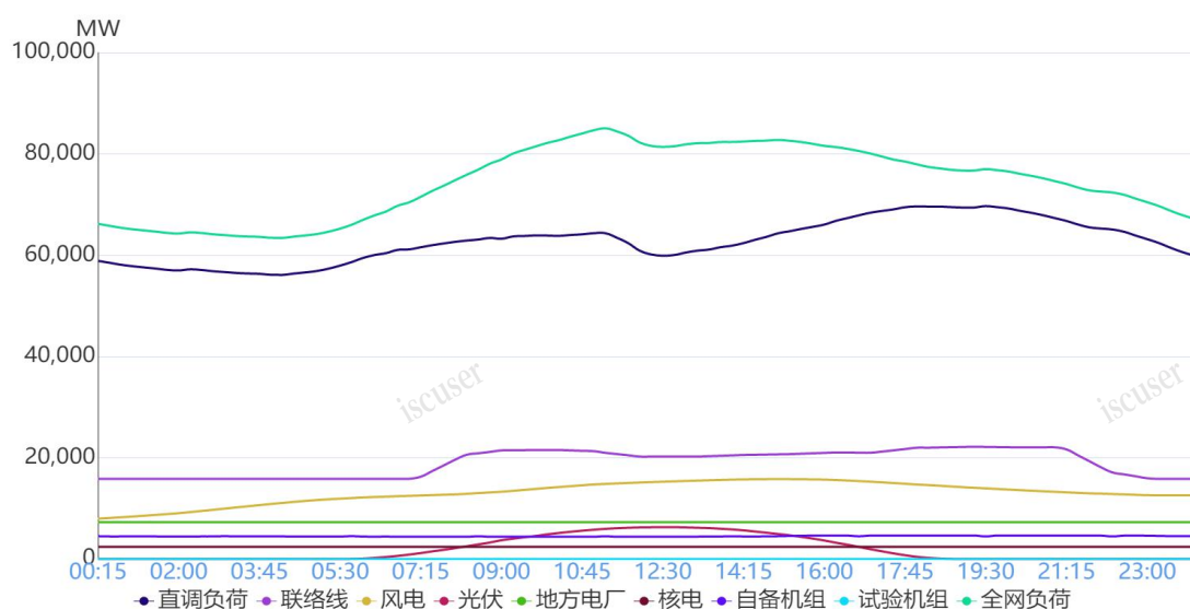
图 1 8月28日负荷及电源出力预测情况
