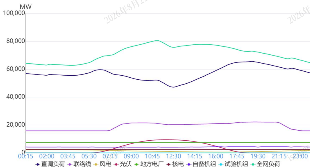
图 1 8 月 30 日负荷及电源出力预测情况
