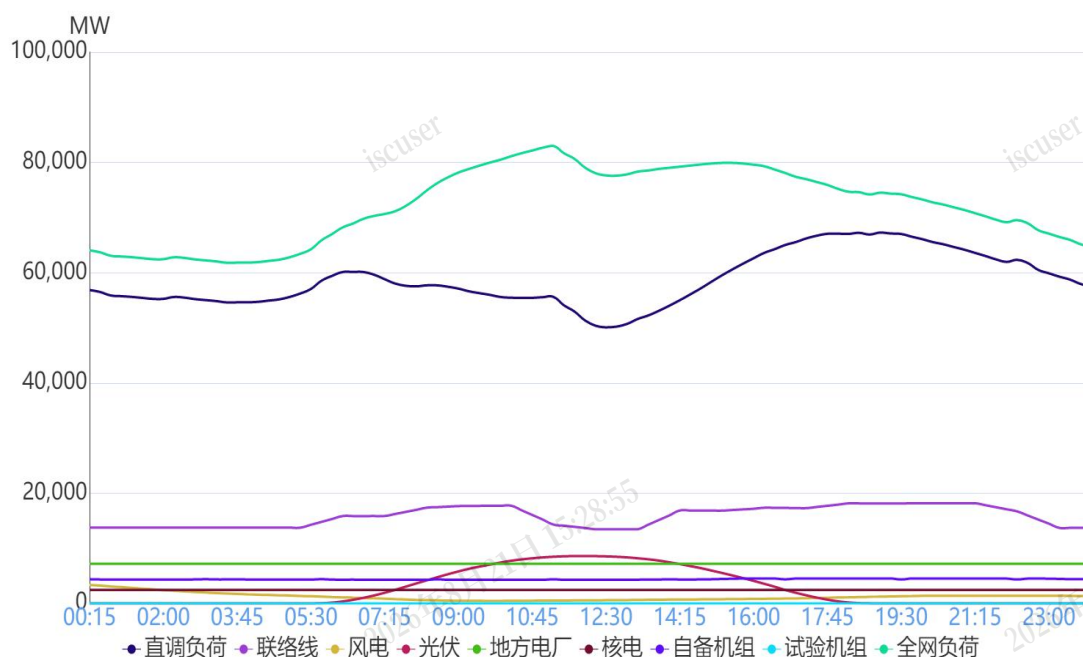
图 1 9月1日负荷及电源出力预测情况
