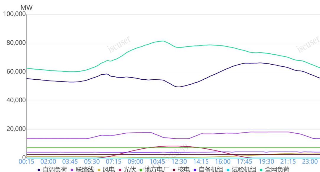
图 1 9月2日负荷及电源出力预测情况
