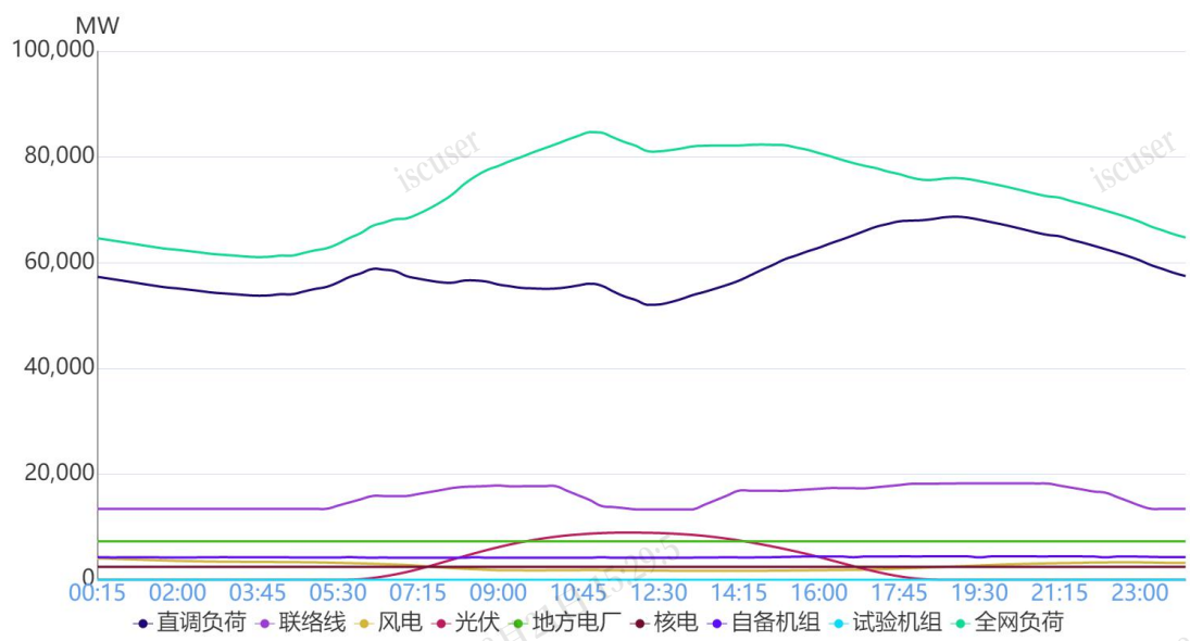
图 1 9月3日负荷及电源出力预测情况
