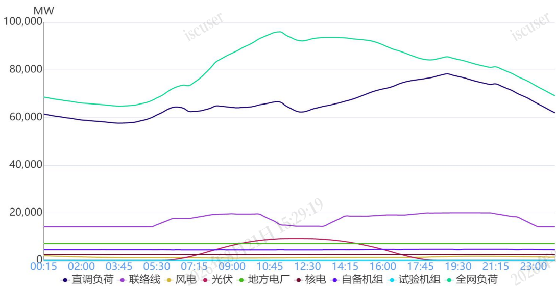
图 1 9月6日负荷及电源出力预测情况
