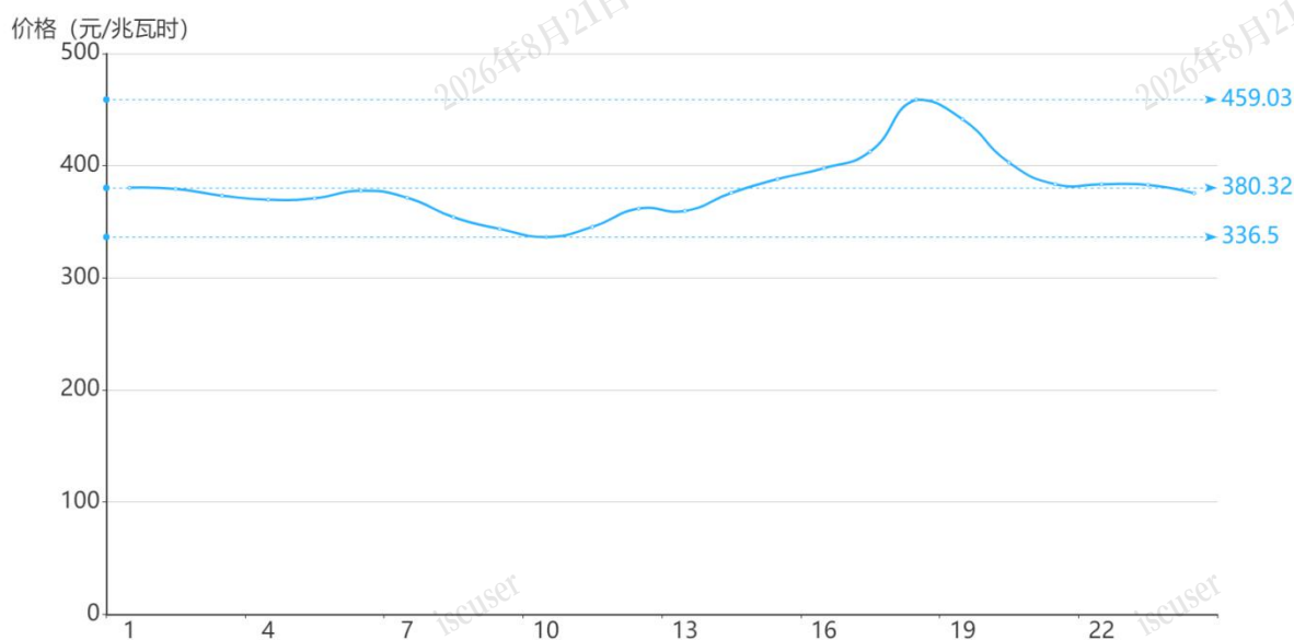
图3 9月9日实时市场用电侧价格
