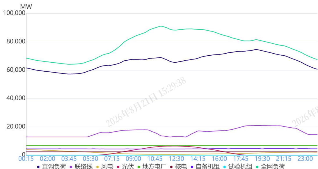
图1 9月10日负荷及电源出力预测情况
