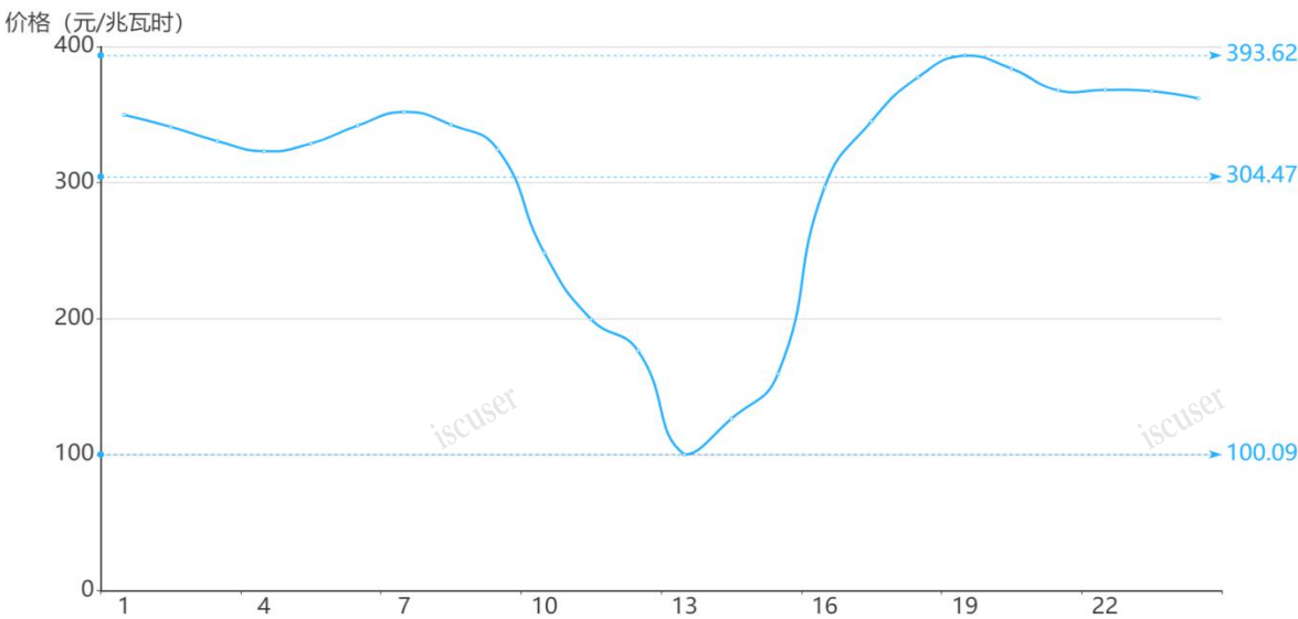
图 3 9 月 13 日实时市场用电侧价格
