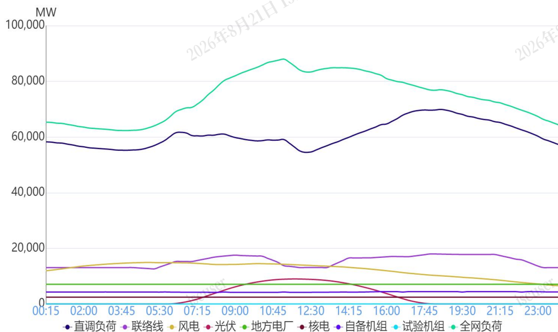
图 1 9月20日负荷及电源出力预测情况
