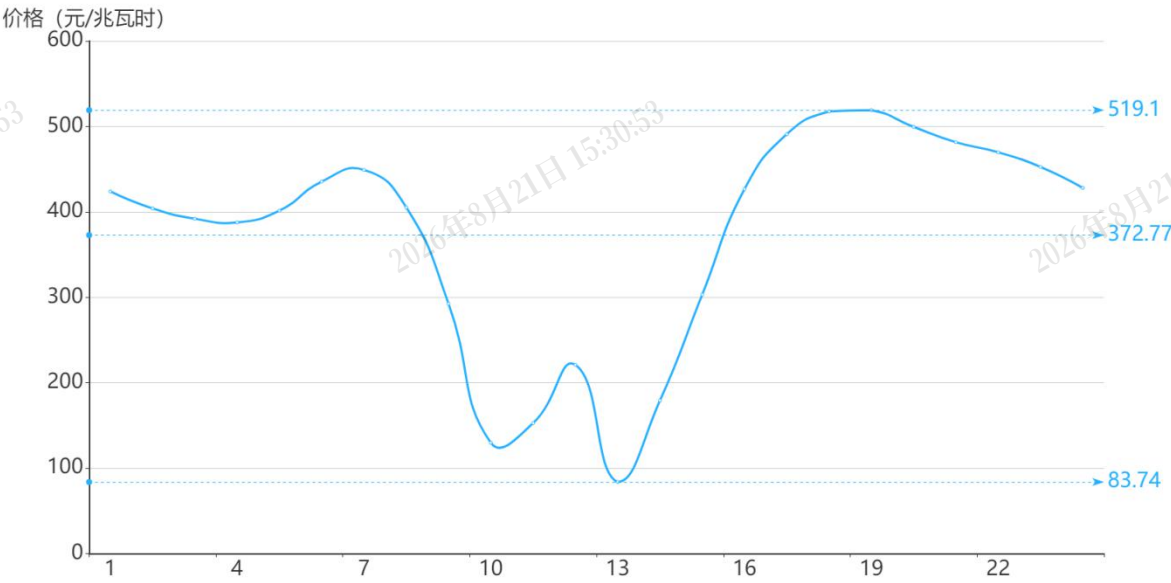
图 2 9 月 22 日日前市场用电侧价格
