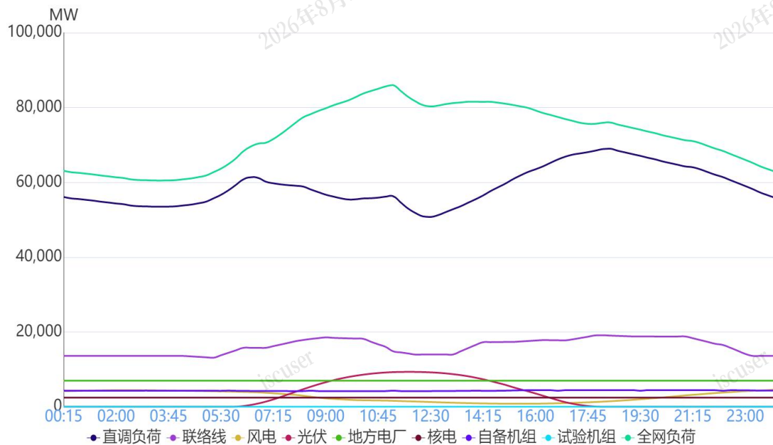
图 1 9月22日负荷及电源出力预测情况
