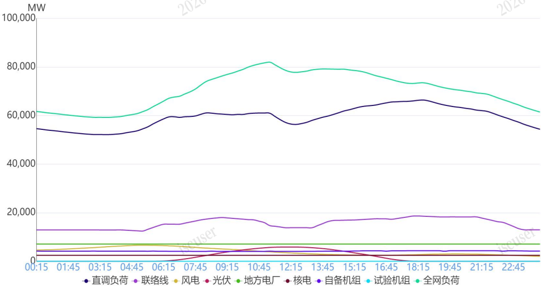
图 1 9月23日负荷及电源出力预测情况
