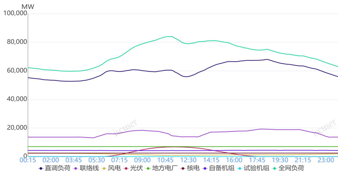
图1 9月26日负荷及电源出力预测情况
